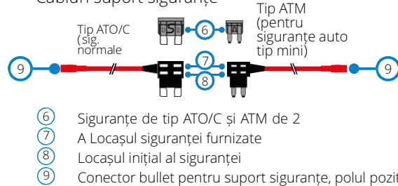
Cabluri suport siguranțe
