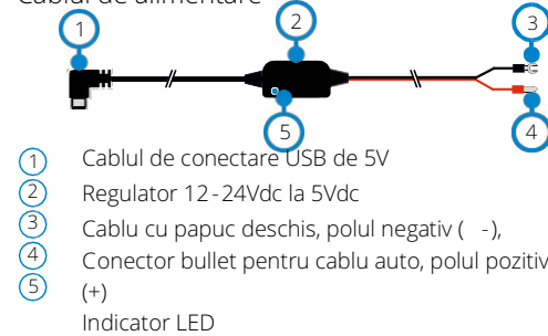
Cablul de alimentare
